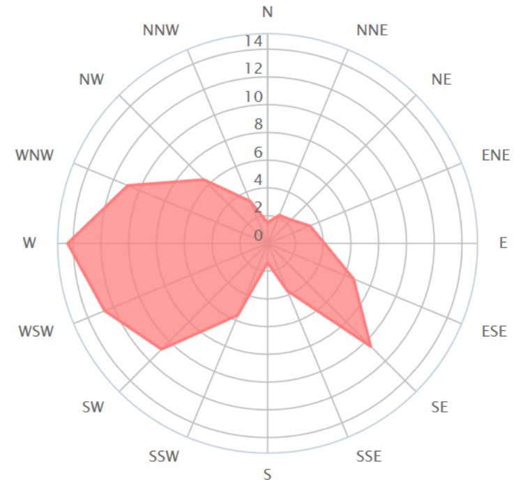
Windrichtungsverteilung in % Juli
